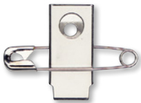
B-023 Metallklammer mit Sicherheitsnadel, drehbar, zum Vernieten, Lochdurchmesser 5 mm, ca. 10 x 25 mm
